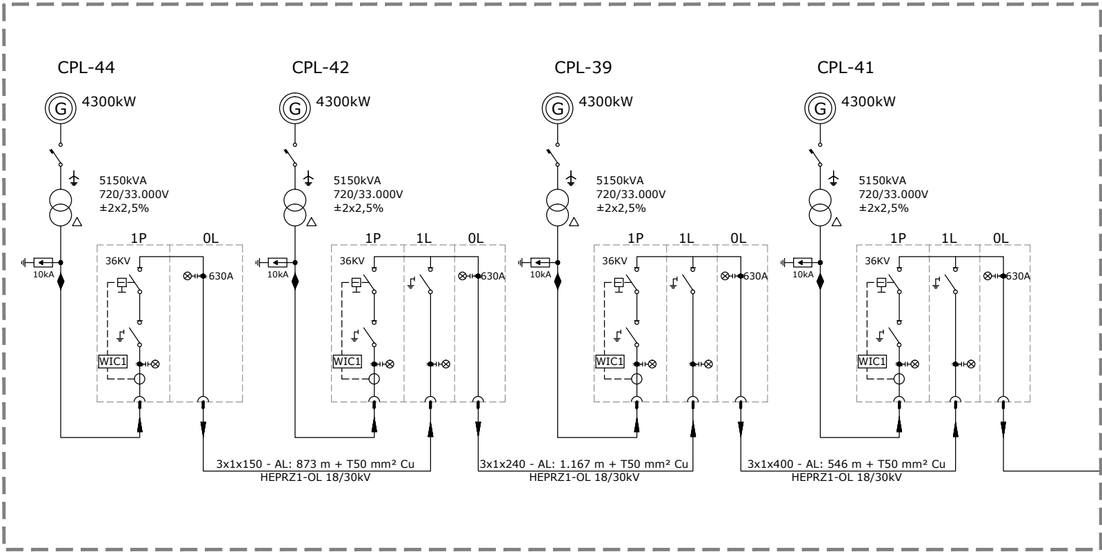
P.E. CAMPO LINDO. CIRCUITO 3
